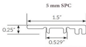
T-MOLD
