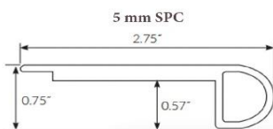
FLUSH STAIRNOSE
